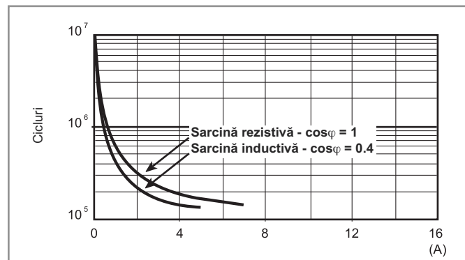
F 58 - Durata de viață electrică (C.A.) v curenul de contact Releu cu 4 contacte
